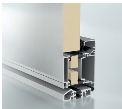
Wypełnienie pokrywające skrzydło z jednej strony, widok z zewnątrz
