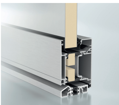
Wypełnienie z widoczną ramą skrzydła, widok z zewnątrz
